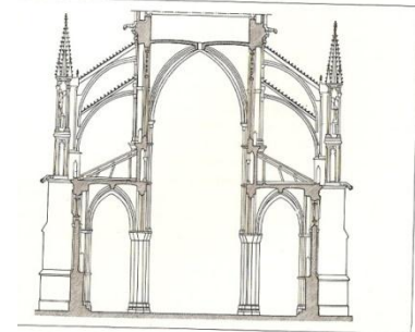
Corte
